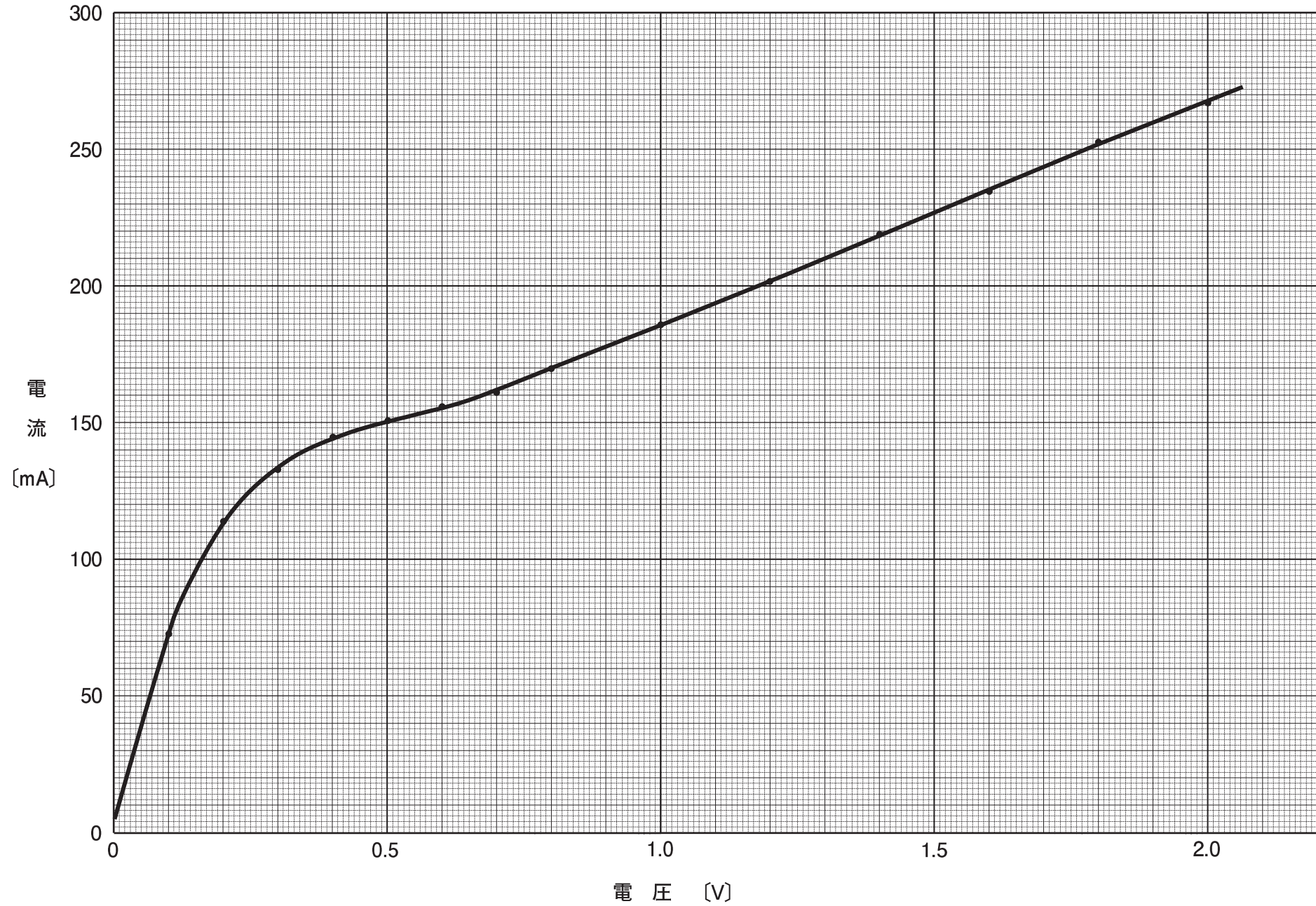
図8. 豆電球にかかる電圧と流れる電流の関係
